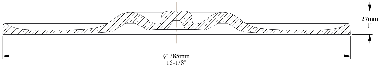
SECTION A-A SCALE 1:2
