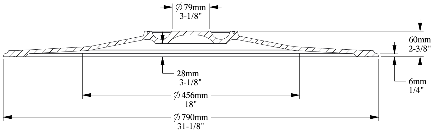
SECTION A-A SCALE 1:5
